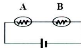
Κύκλωμα 2
